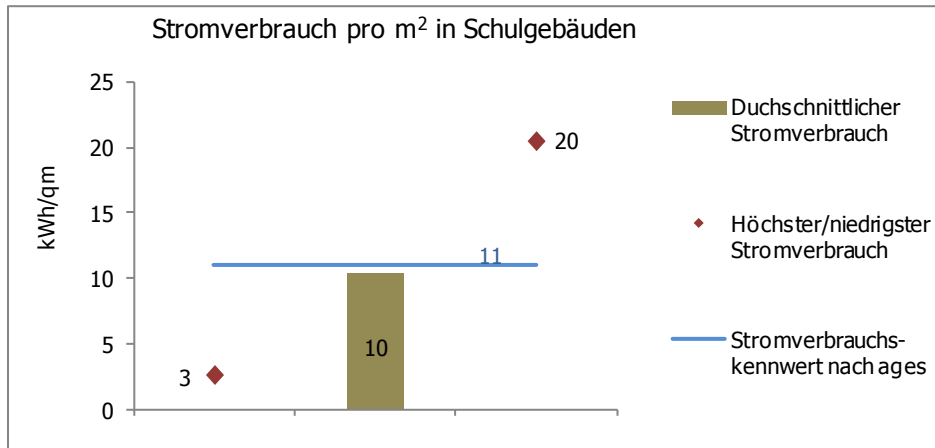
Abbildung 53: Benchmark Stromverbrauch Schulgebäude
