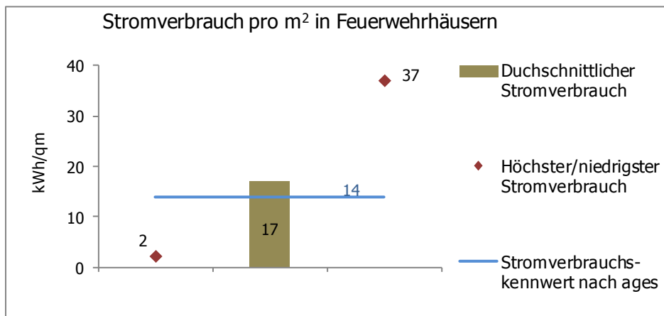
Abbildung 50: Benchmark Stromverbrauch Feuerwehrhäuser
