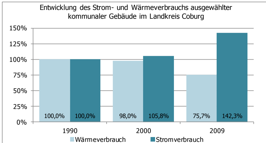
Abbildung 44: Entwicklung Energieverbrauch kommunaler Liegenschaften 1990 -2009
