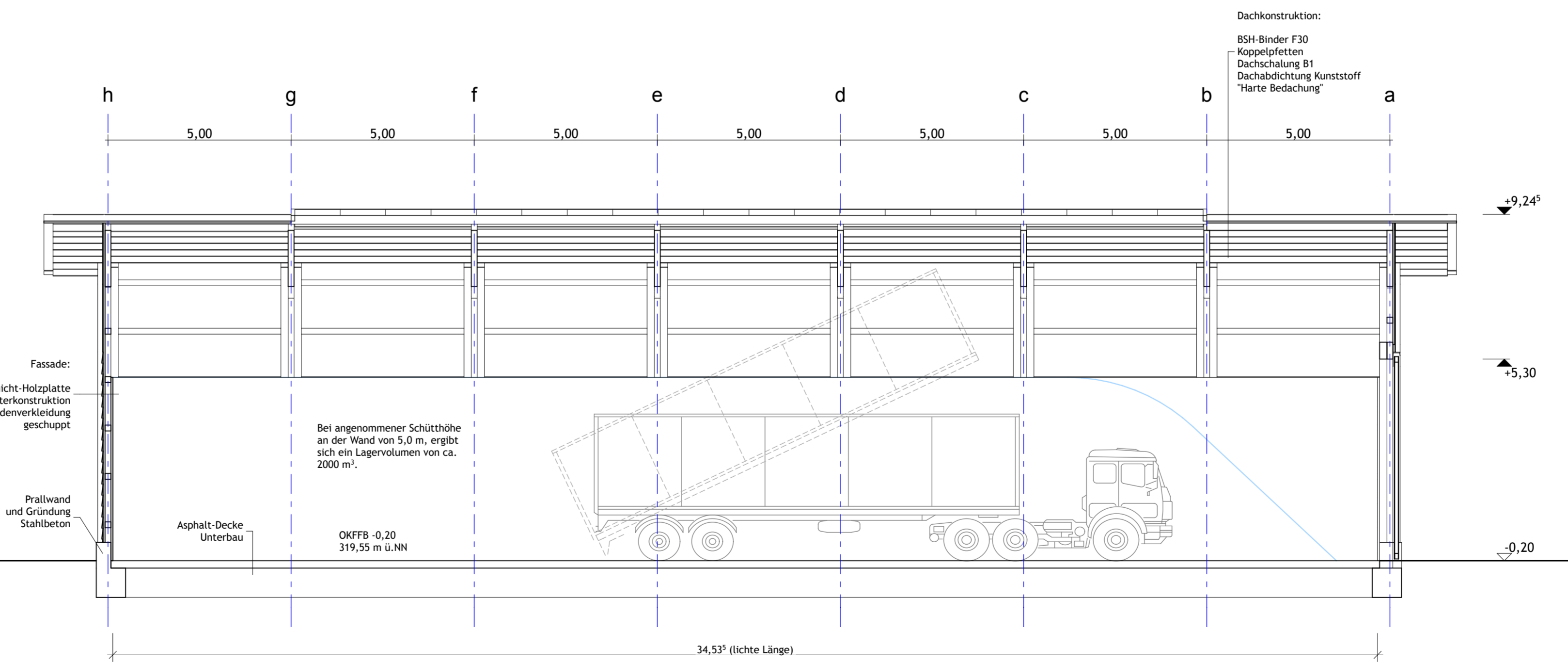
SCHNITT CC 1:100
